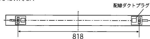
取付面見上げ図
