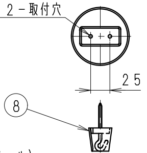
取付面寸法図
