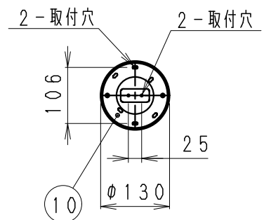
取付面寸法図
