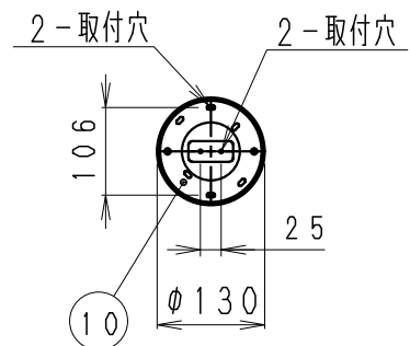
取付面寸法図
