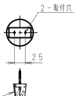
取付面寸法図
