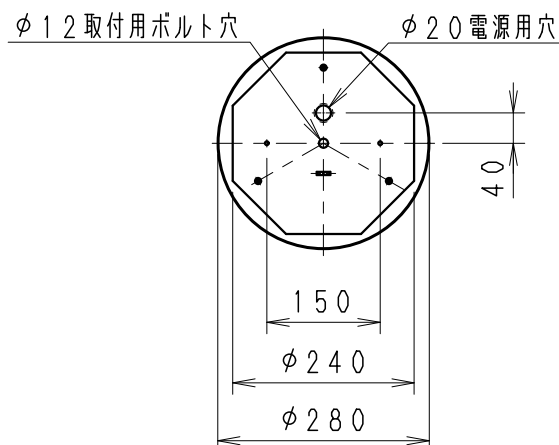
取付面寸法図 (S = 1 / 10)
