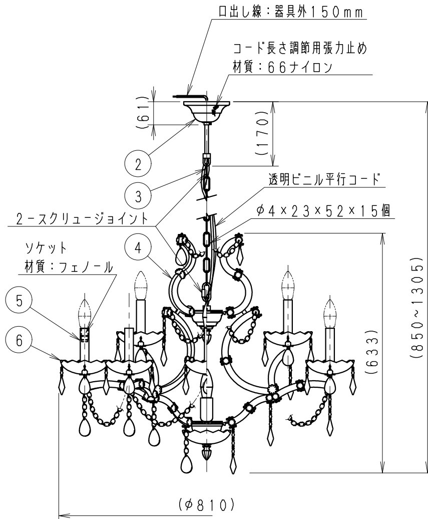
取付面寸法図 S = 1/5
