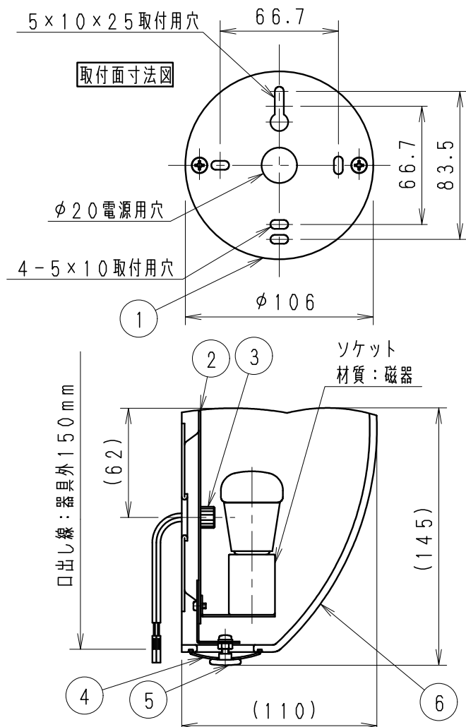
取付位置寸法
