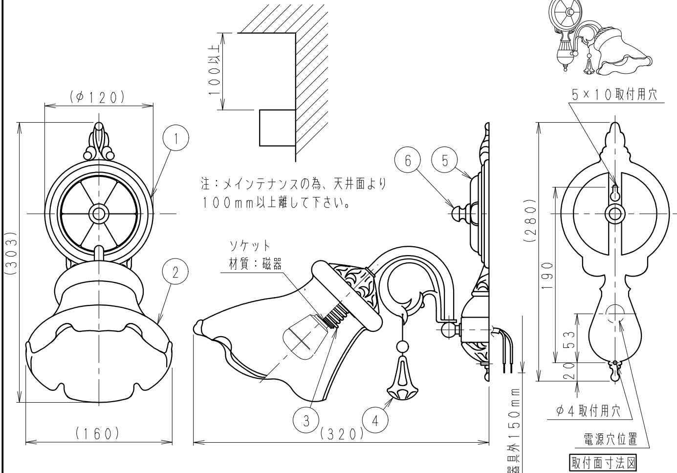
取付位置寸法
