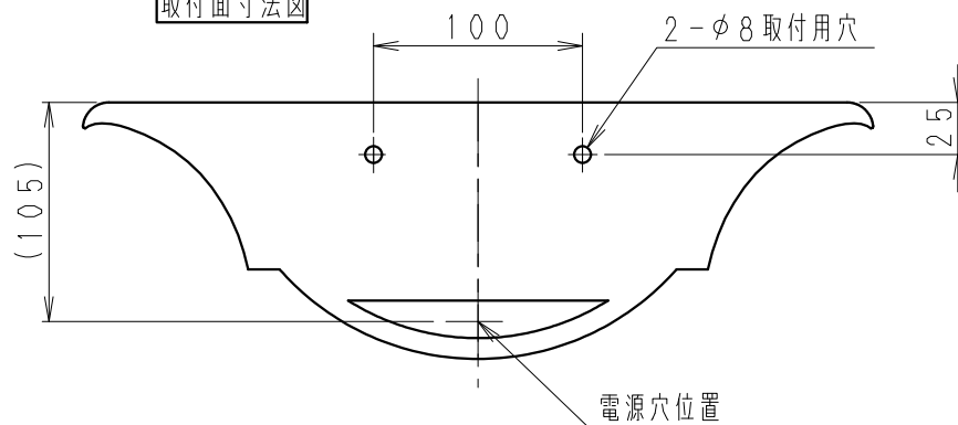
取付面寸法図
