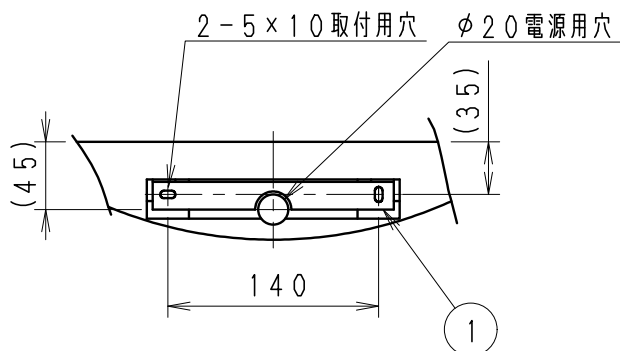
取付面寸法図
