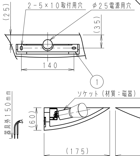
取付面寸法図
