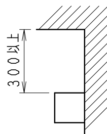
取付位置寸法
