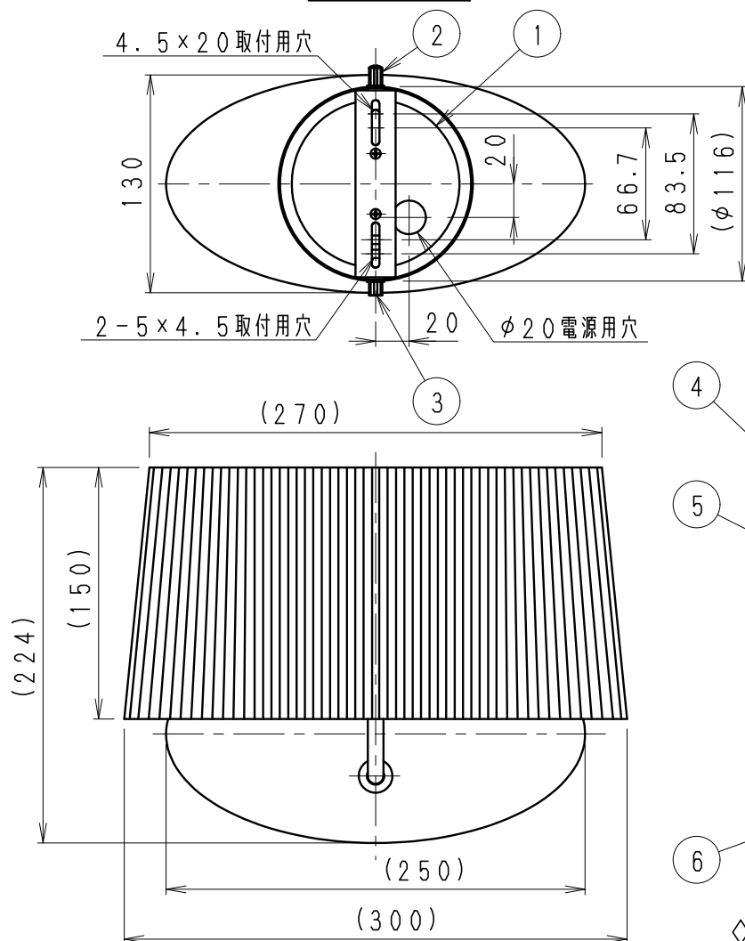
A矢取付面寸法図
