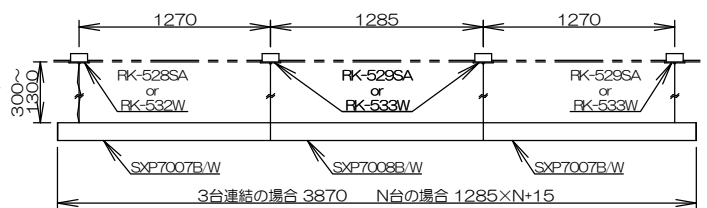
ペンダント取付寸法
