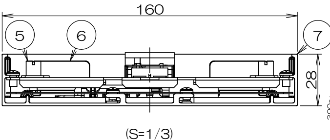
ペンダント取付寸法
