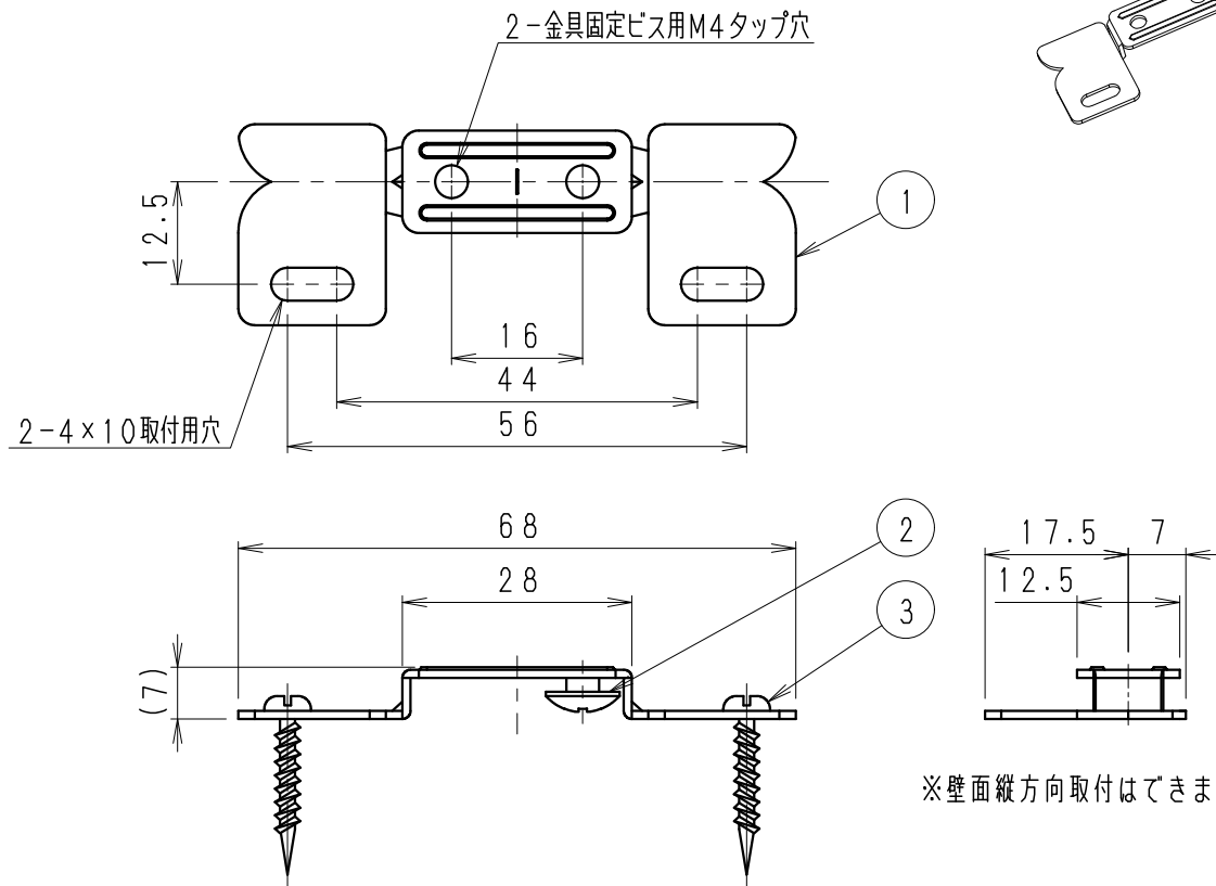
適合器具組み合わせ図 S = 1 / 2
