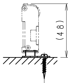
適合器具組み合わせ図 S = 1 / 2
