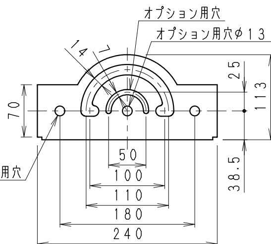
取付寸法
