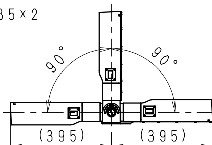
首振可能範囲 (S=1/15)
