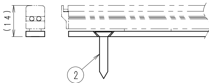
ユニット取付図
