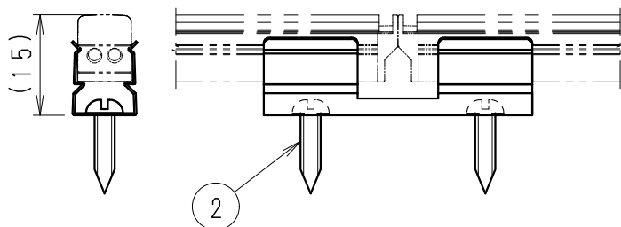
ユニット取付図 (縮尺1/1)
