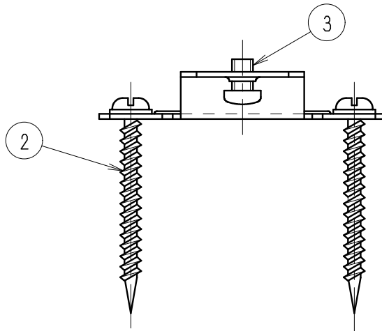
本体組立図 (1/3)
