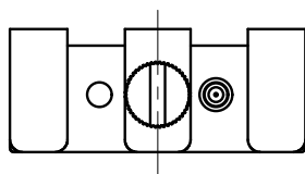
A矢視図 (1/1)
