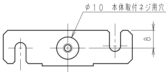
本体組合図 (1/3)
