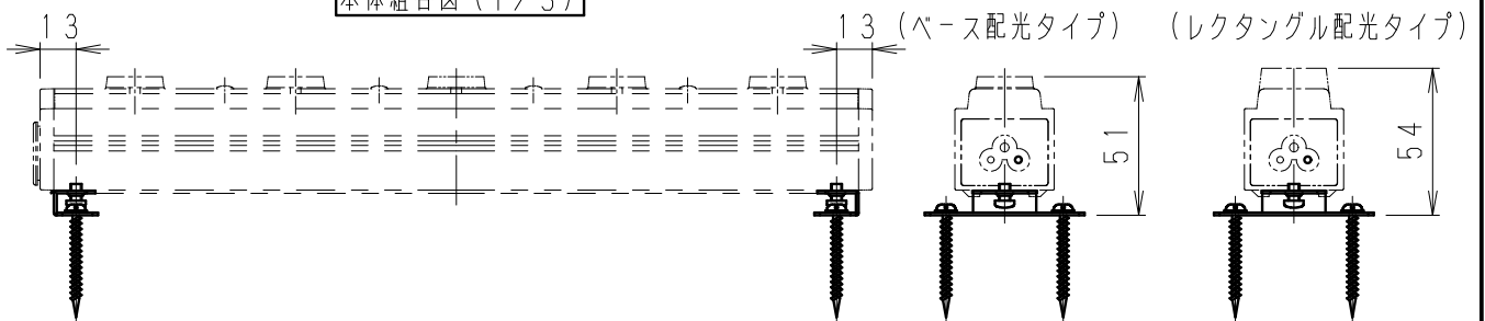
本体組合図 (1/3)
