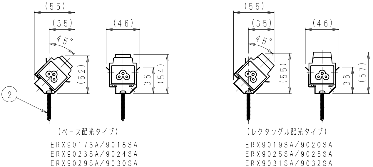
本体組合図 (1/3)
