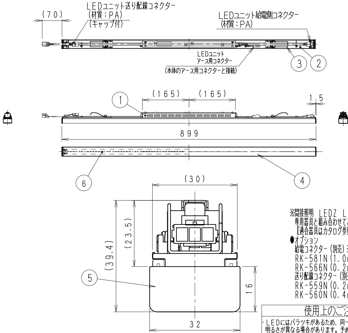
側面図 1/1
