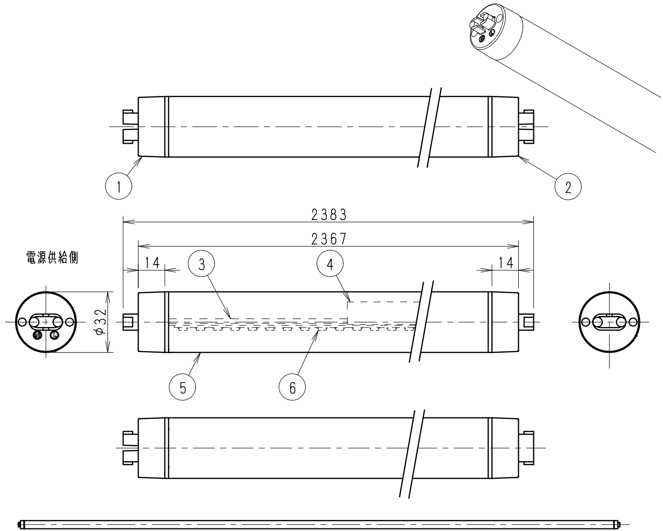
全体図 1/15
