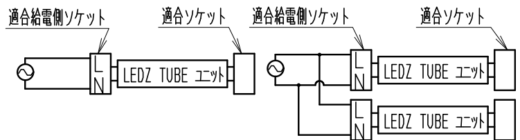
1灯用結線図
