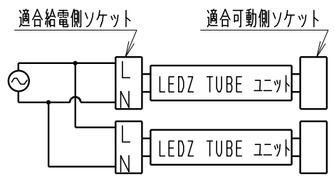
2灯用結線図
