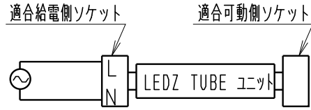
1灯用結線図
