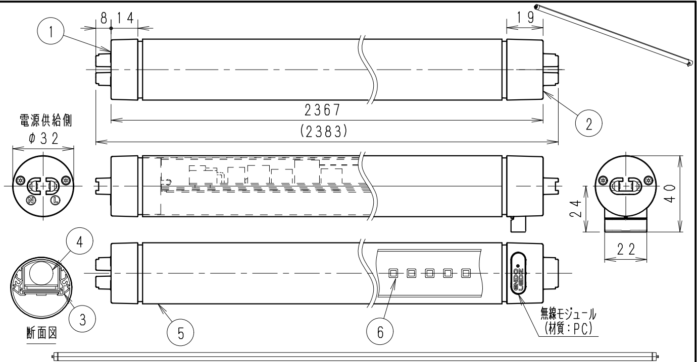
全体図 1/15
