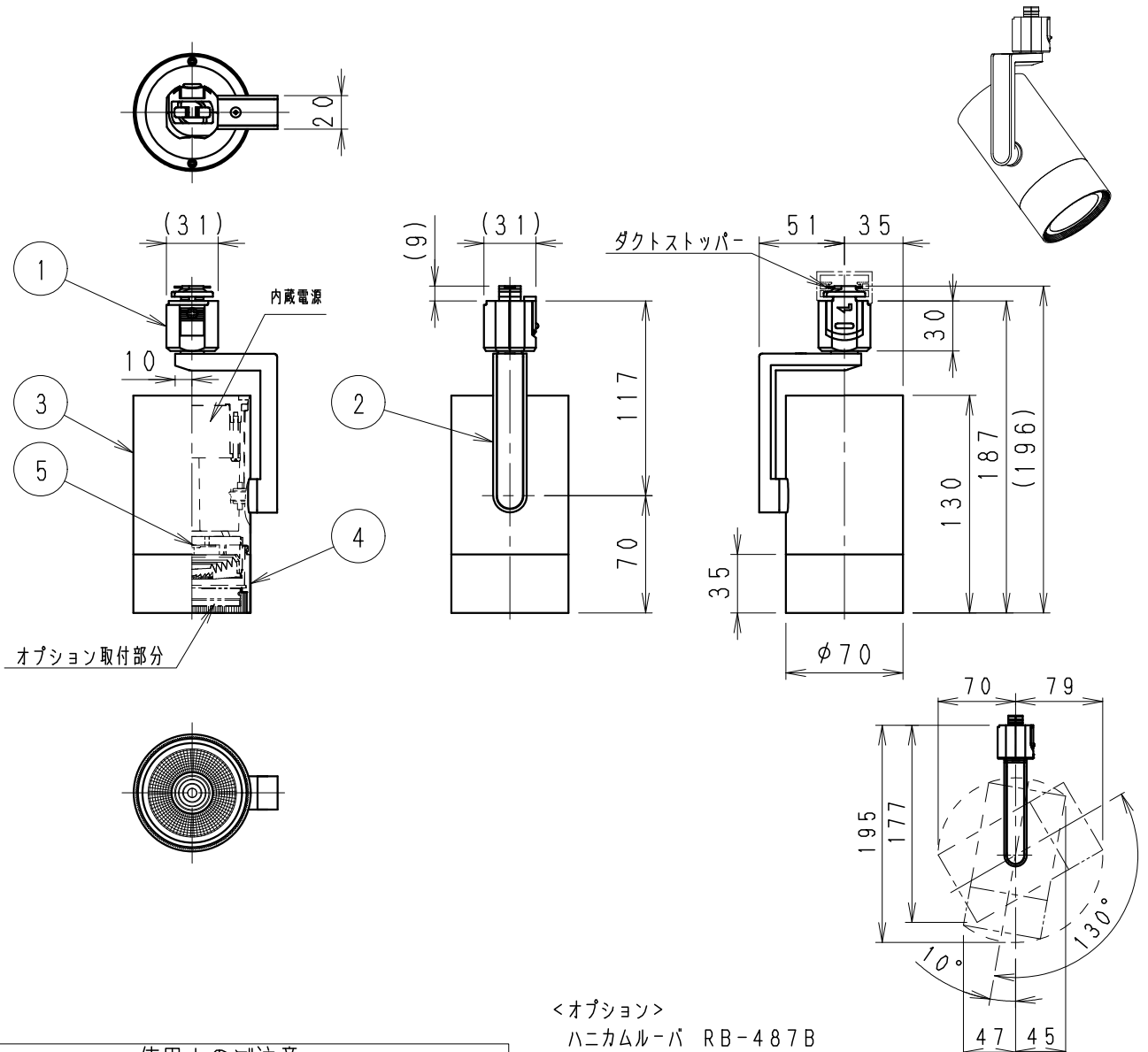
灯具可動範囲図示
