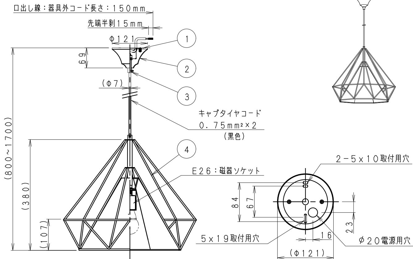
取付板寸法詳細
