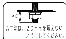
取付ボルトの器具内寸法
