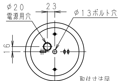
取付寸法図 A矢視図(1/6)
