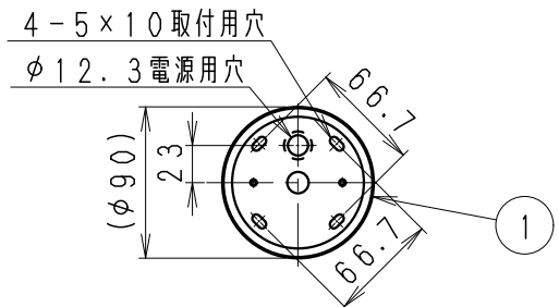
取付面寸法
