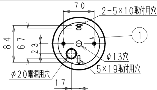
取付寸法図 (A-A)
