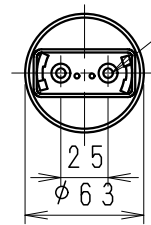
取付面寸法図
