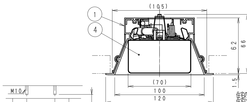
断面図 (S=1/2)
