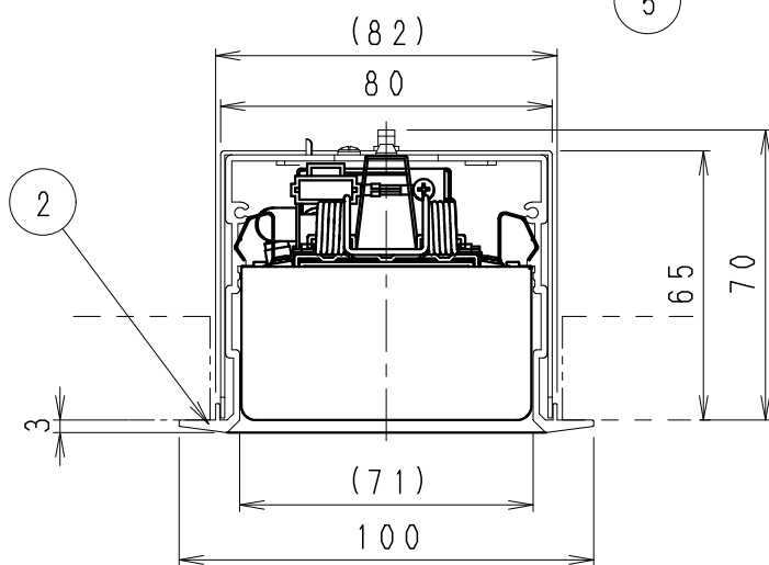
断面図 (S=1/2)
