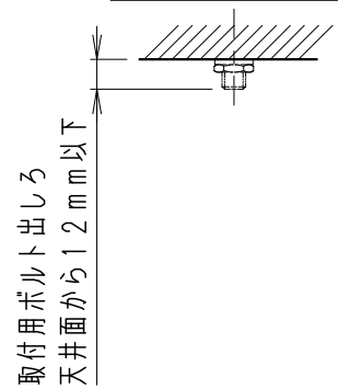
取付用ボルト取付寸法
