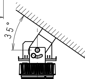
傾斜天井取付範囲図 S=1/10
