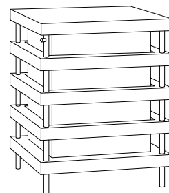
4-φ12ボルト取付用穴兼水抜用穴 (ボルト未使用可能)
