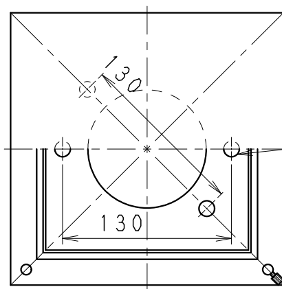
4-φ12ボルト取付用穴兼水抜用穴 (ボルト未使用可能)
