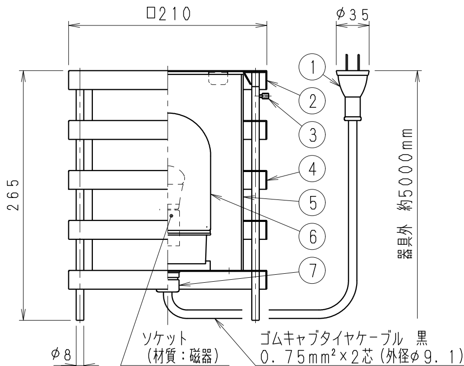
4-φ12ボルト取付用穴兼水抜用穴 (ボルト未使用可能)
