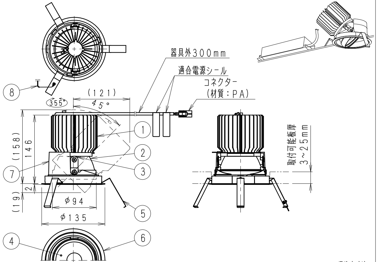
埋込寸法
