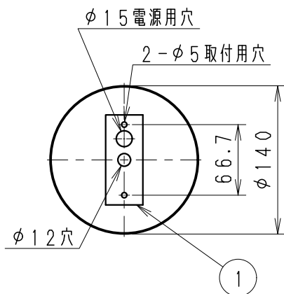
取付面寸法図 S=1/5
