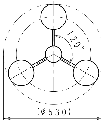
底面図 S=1/12
