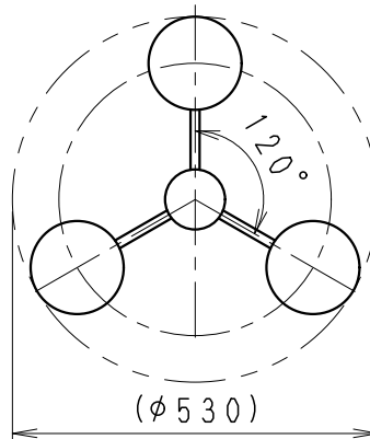
底面図 S=1/12
