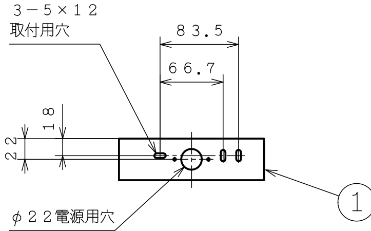
取付面寸法図 (S=1/4)
