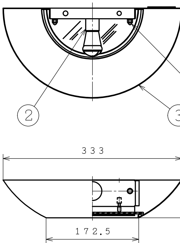
取付面寸法図 (S=1/4)
