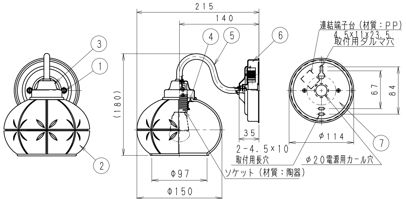
取付面寸法図
