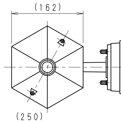
取付位置寸法
