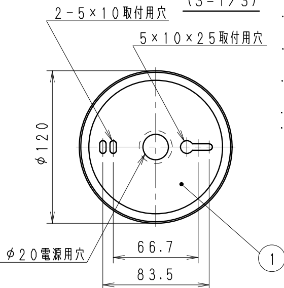
取付面寸法図 (S=1/3)
