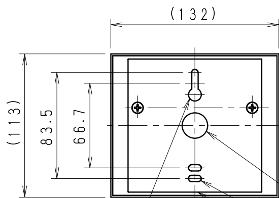
取付面寸法図
