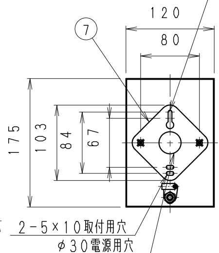
取付寸法図 (A矢視図)
