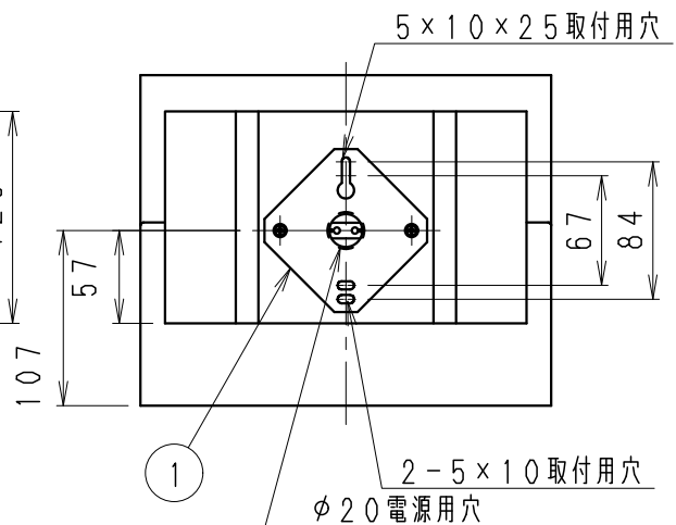
取付寸法図 (A矢視図)
